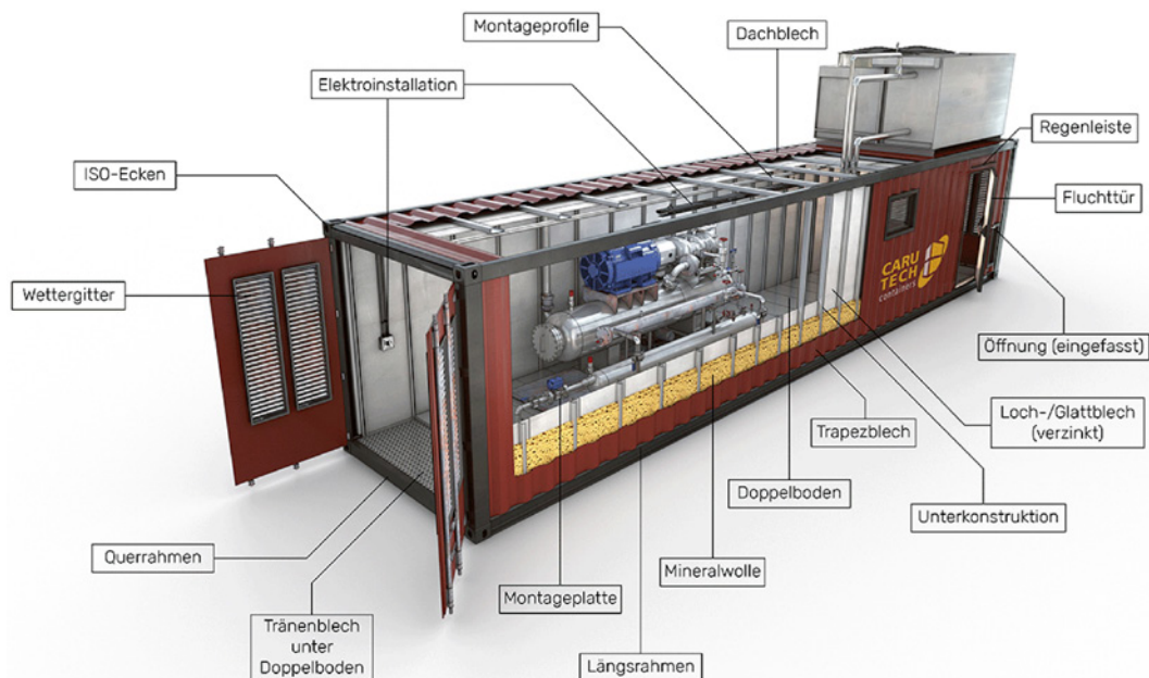
8- 20 ft Basic-Technikcontainer – pulverlackiert –
